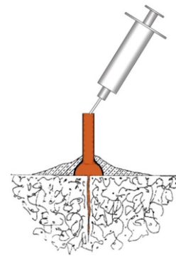
Fig. 2: Consolidación de grieta inyectando resina epoxi
