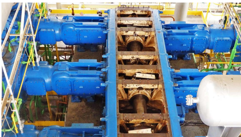
Pormenor do compressor alternativo em processo de manutenção.
